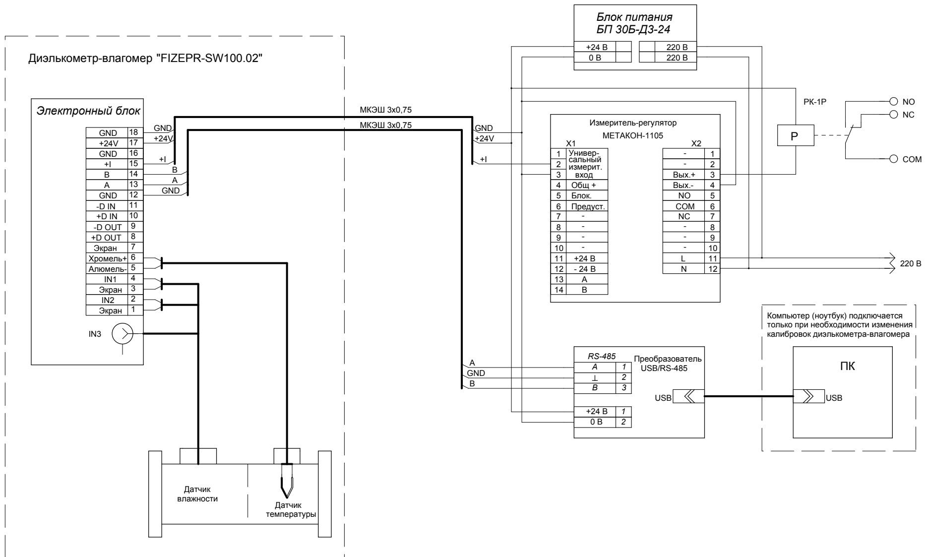
Схема подключения дизелькометра-влажгомера
